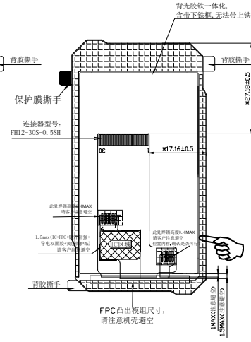
FPC弯折示意图 FPC弯折出货
